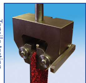
Tensile testing
